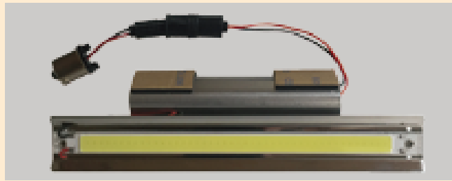
バス用LED路肩灯
